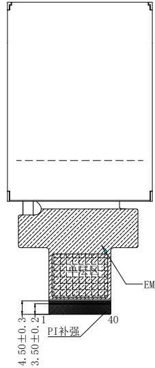
FPC展开参考图
