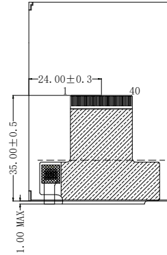
FPC弯折参考图
