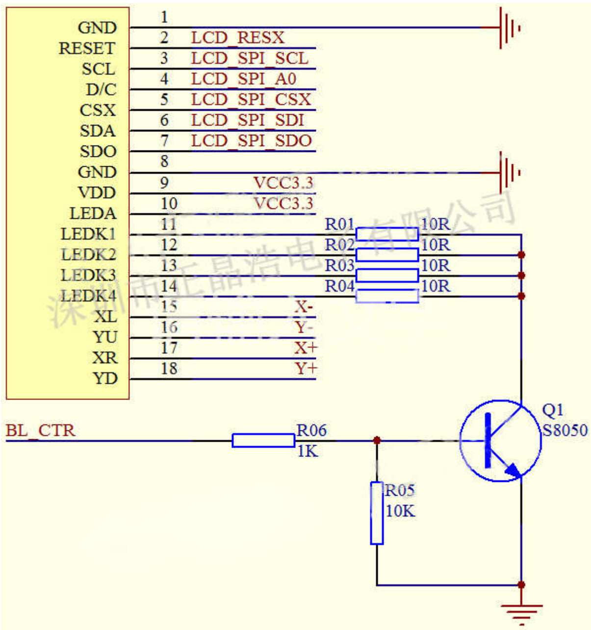
附图 6-1: 显示屏 YT240S030_4 线-SPI 串口参考应用电路
