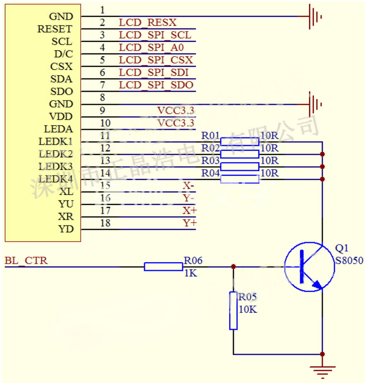
附图 6-1: 显示屏 YT240S010_4 线-SPI 串口参考应用电路
