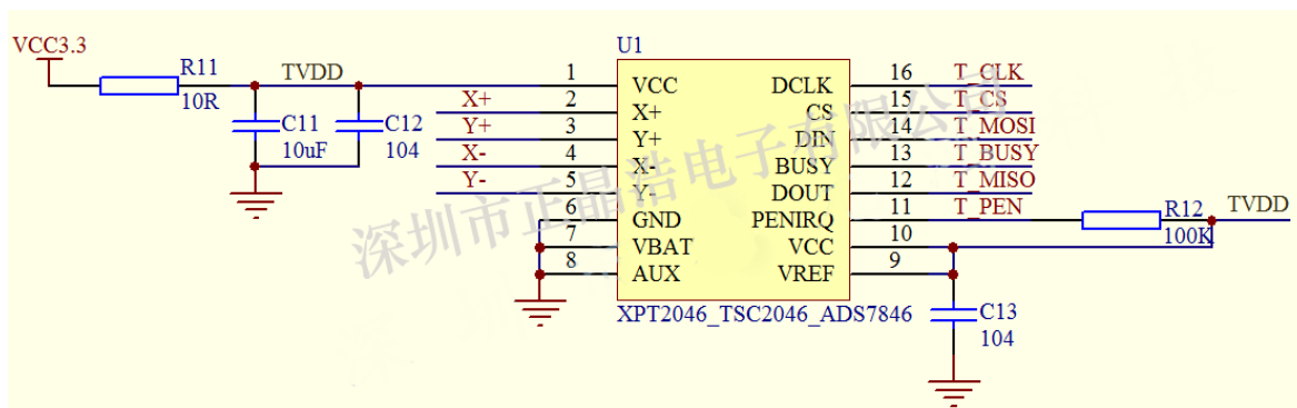
附图 6-2: 触摸屏参考应用电路
