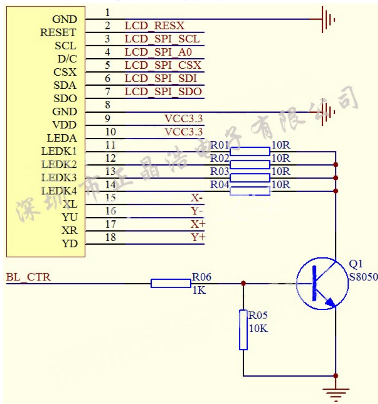
附图 6-1: 显示屏 YT280S030_4 线-SPI 串口参考应用电路
