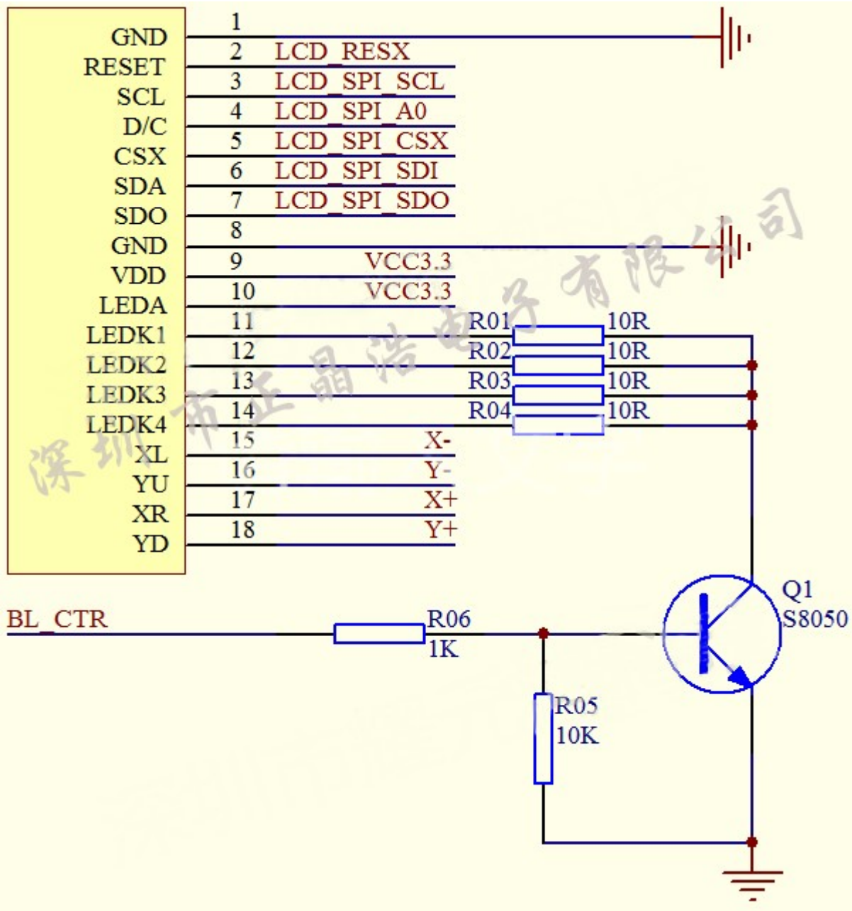
附图 6-1: 显示屏 YT280L030_4 线-SPI 串口参考应用电路
