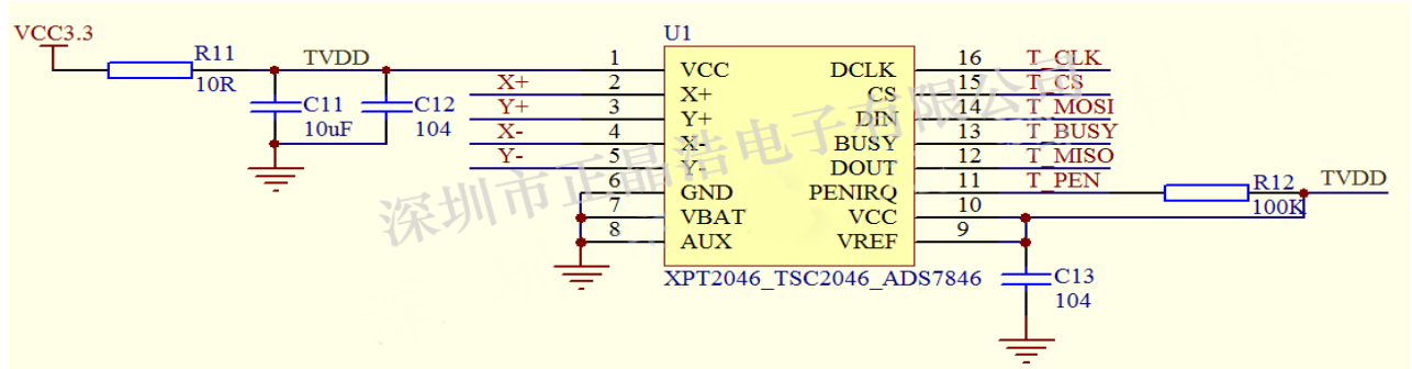
附图 6-2: 触摸屏参考应用电路
