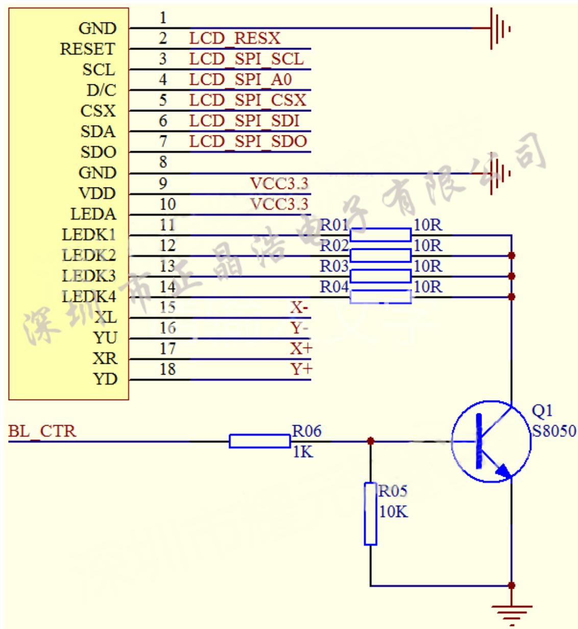
附图 6-1: 显示屏 YT280S010_4 线-SPI 串口参考应用电路
