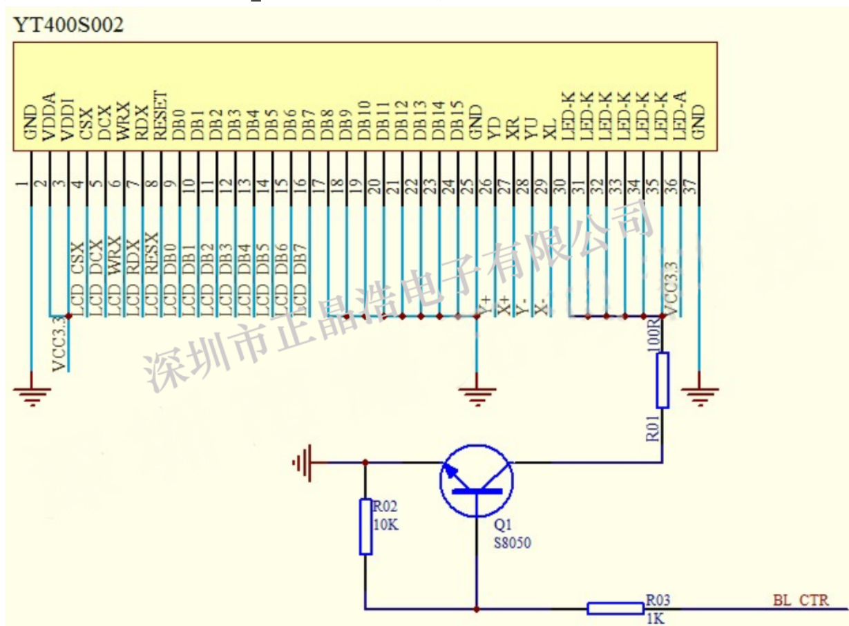
附图 6-3: 触摸屏参考应用电路
