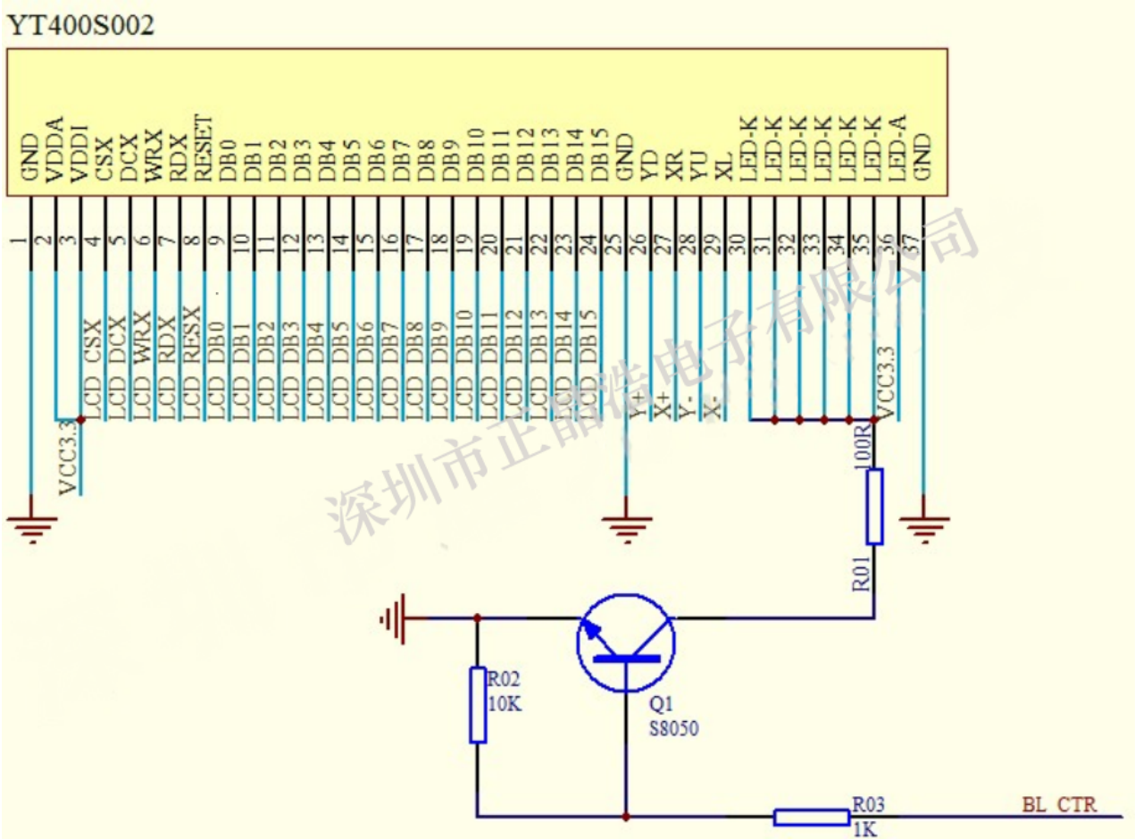
附图 6-1: 显示屏 YT400S002_16 位并口参考应用电路
