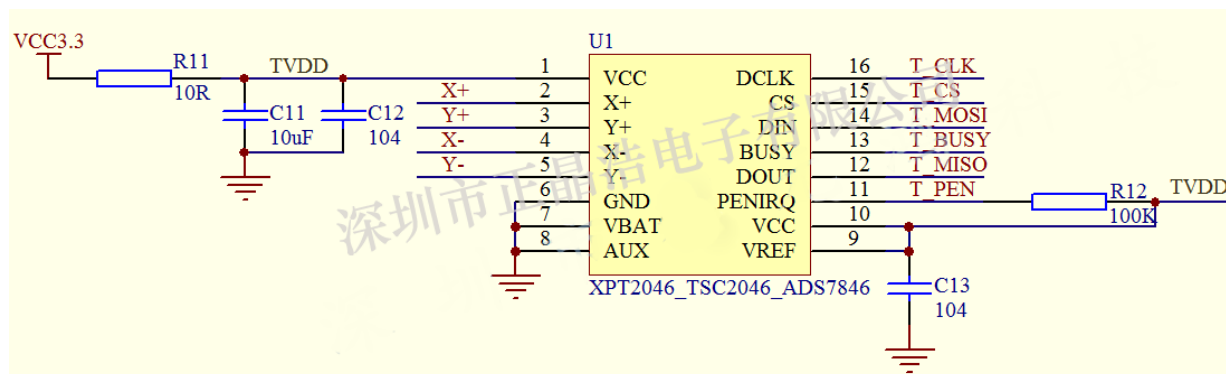
附图 6-3: 触摸屏参考应用电路
